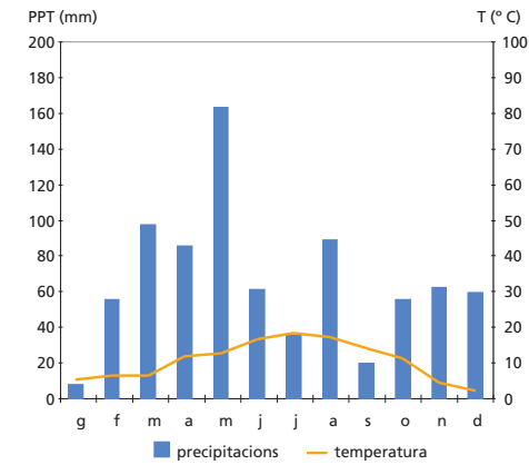
Diagrama ombrotèrmic. Val d'Aran. 2007
